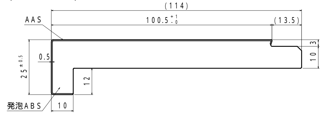
縦枠(100タイプ) 合板なし
