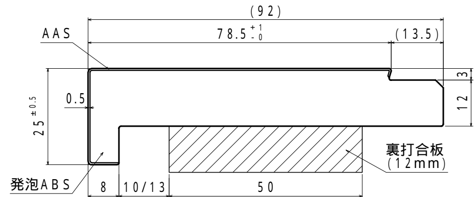
上下枠(80タイプ) 合板付き溝10 / 溝13
