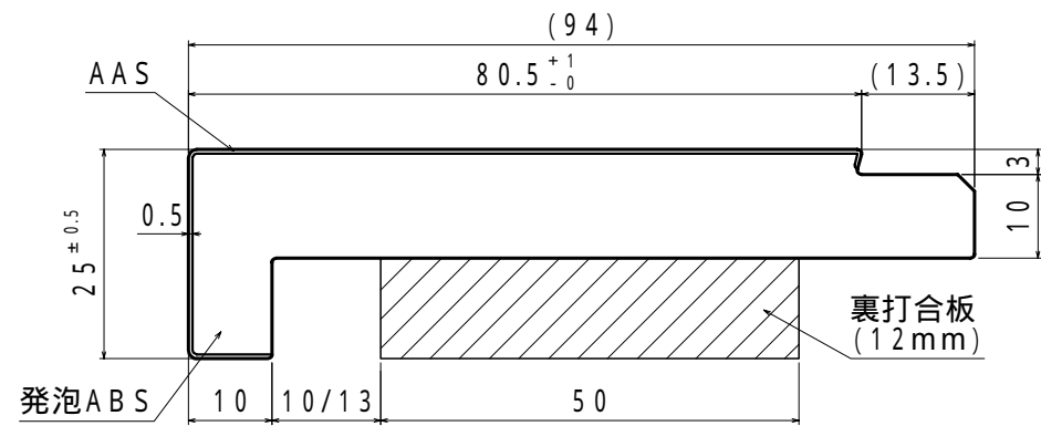
縦枠(80タイプ) 合板付き溝10 / 溝13
