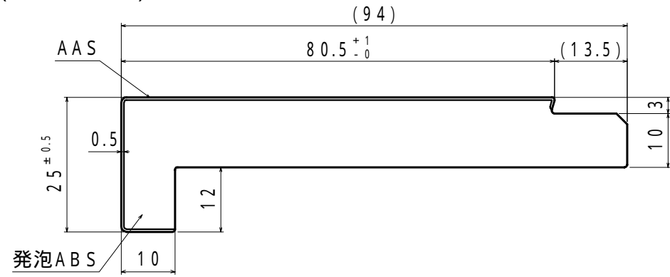
縦枠(80タイプ) 合板なし
