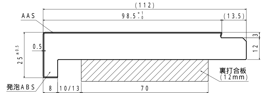
上下枠(100タイプ) 合板付き溝10 / 溝13
