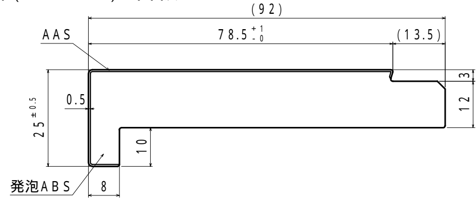
上下枠(80タイプ) 合板なし
