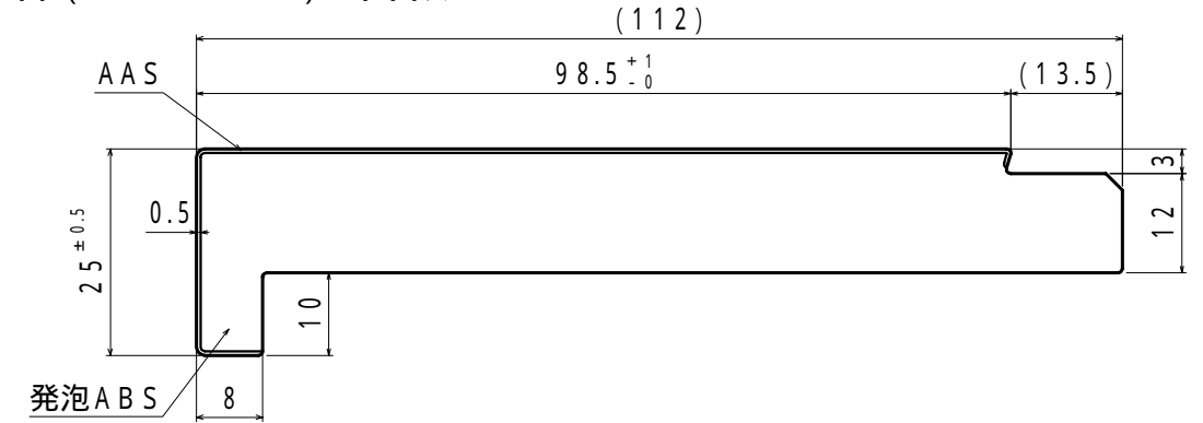
上下枠(100タイプ) 合板なし
