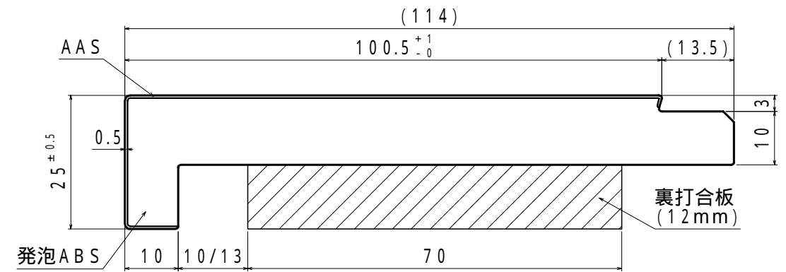
縦枠(100タイプ) 合板付き溝10 / 溝13
